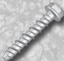
ISA-8~14 二条ねじ
